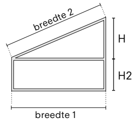
P78 Driehoek plus
